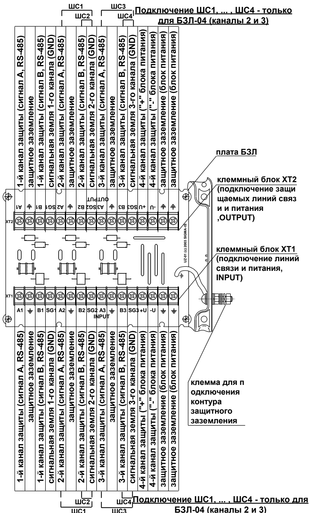
Рис. 3 Плата БЗЛ-01, БЗЛ-04
